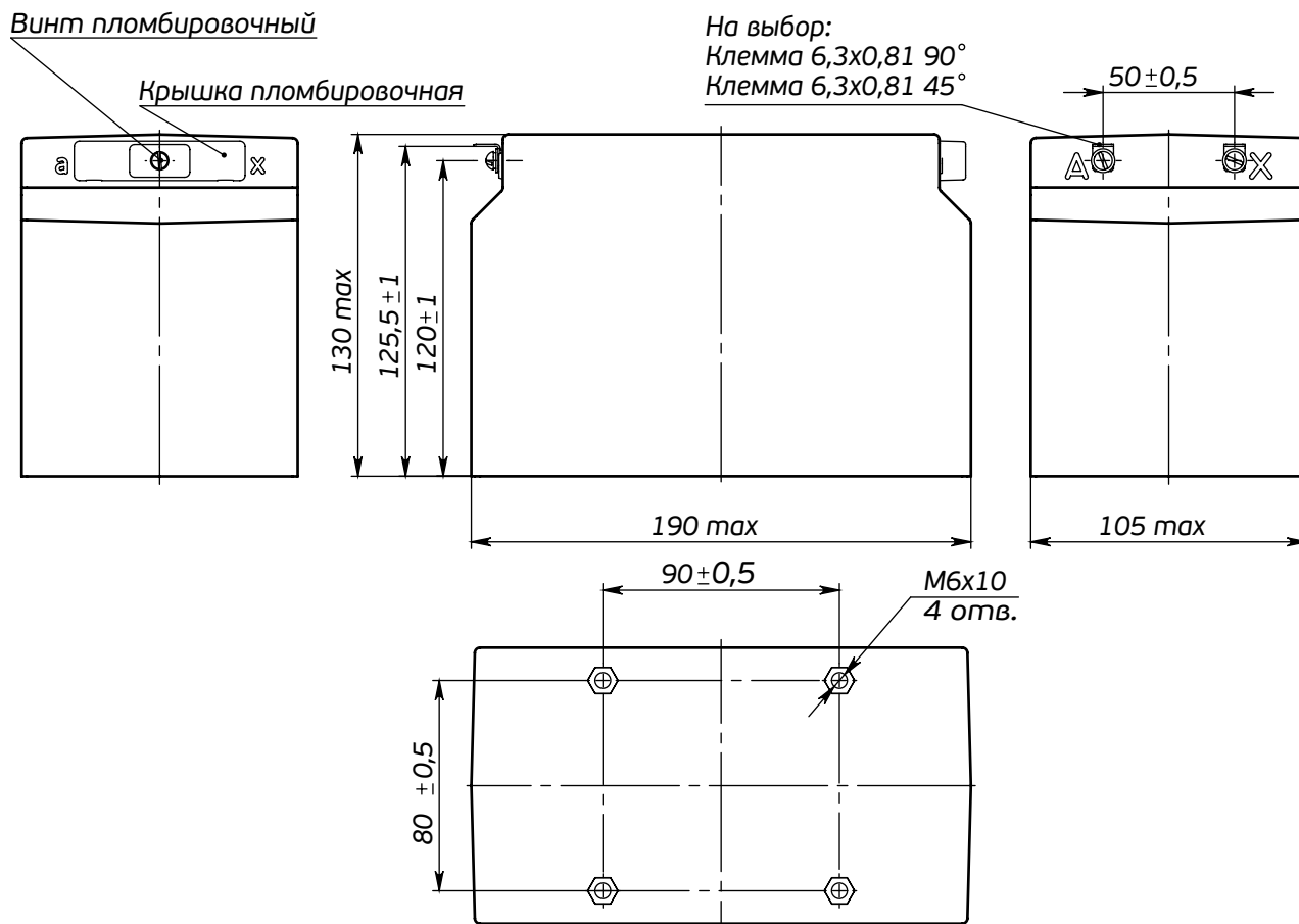
Рис. 1 - Общий вид трансформатора ЗНОЛ-СВЭЛ-0,66
